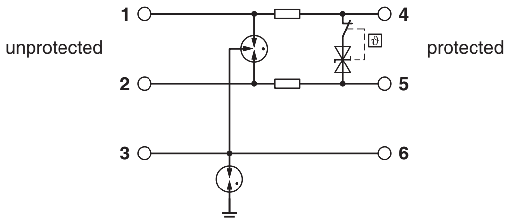
Diagrama eléctrico
