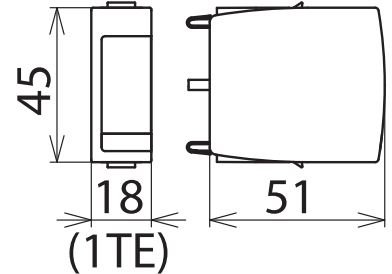
Maßbild DG MOD H PV 750
