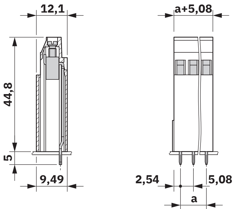
Dessin coté
