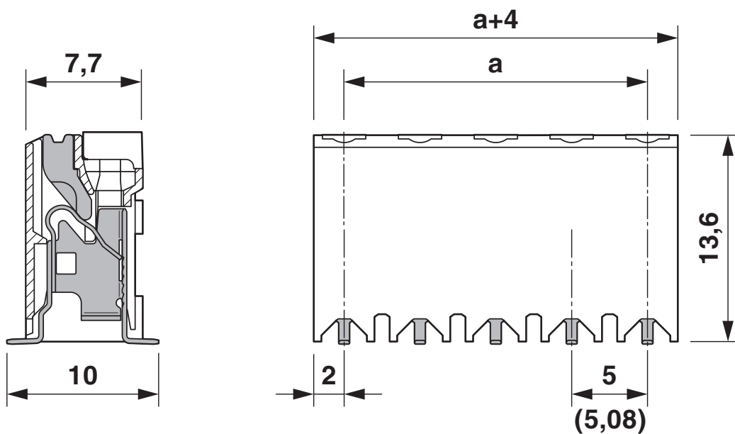
Maßzeichnung
