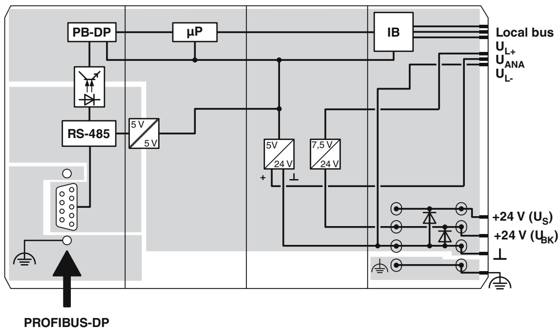
Schéma fonctionnel
