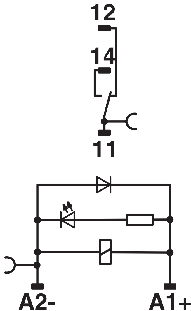
Diagrama eléctrico
