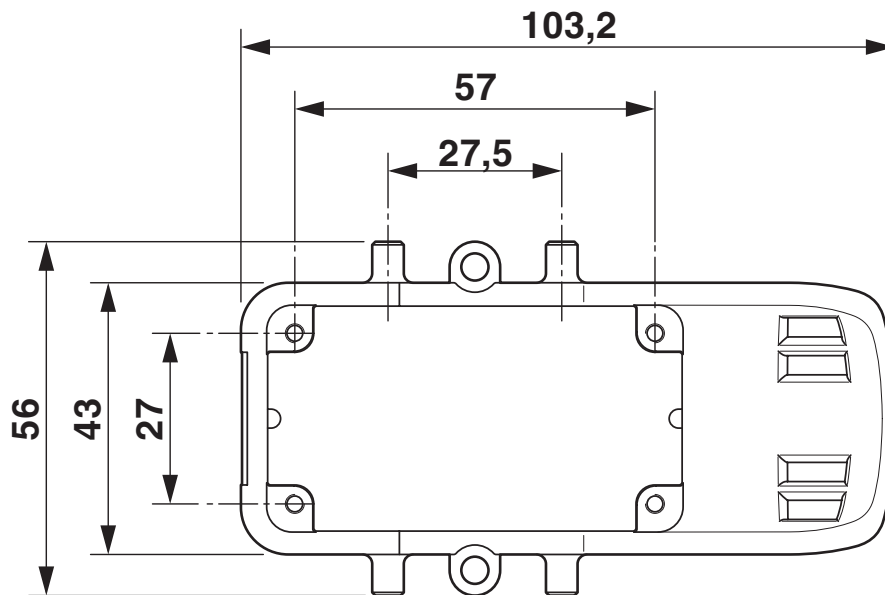
Maßzeichnung
