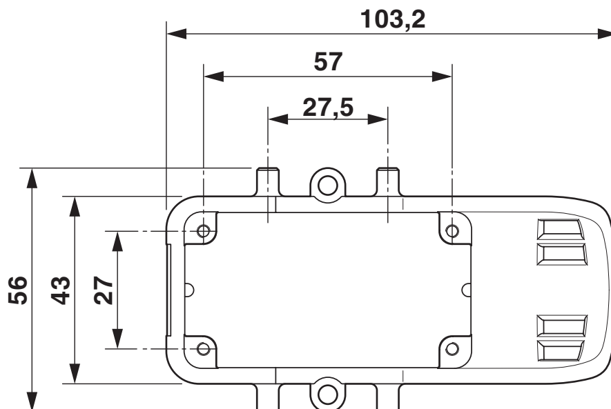
Esquema dimensiones vista desde arriba
