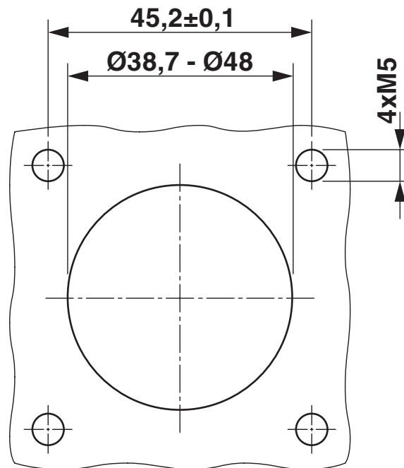
Bohrplan/Lötpadgeometrie
