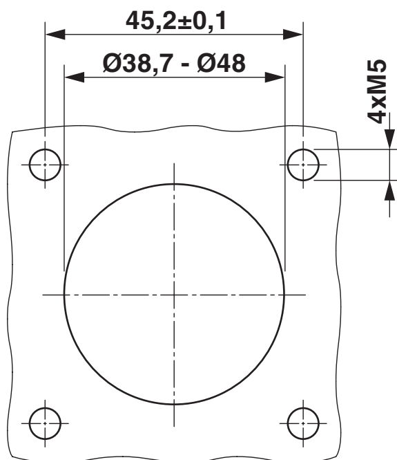
Esquema de taladros/geometría pads soldadura
