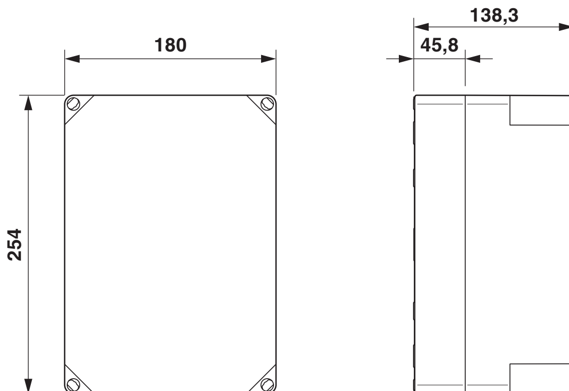
Dessin coté
