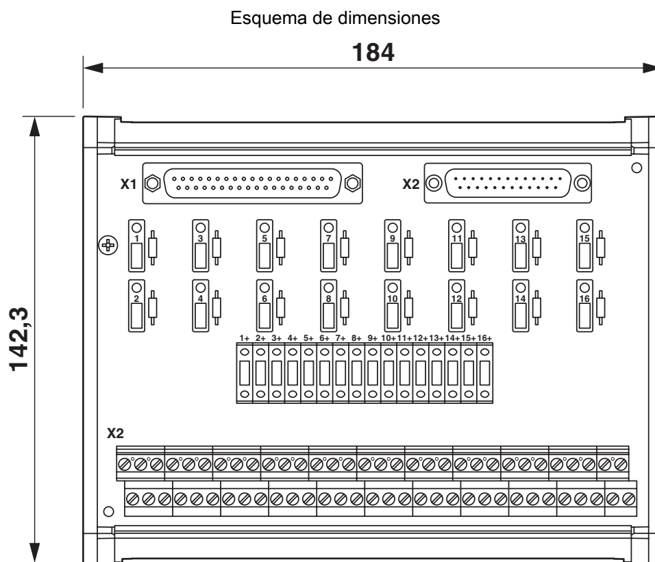
Esquema de dimensiones para versión para zurdos
