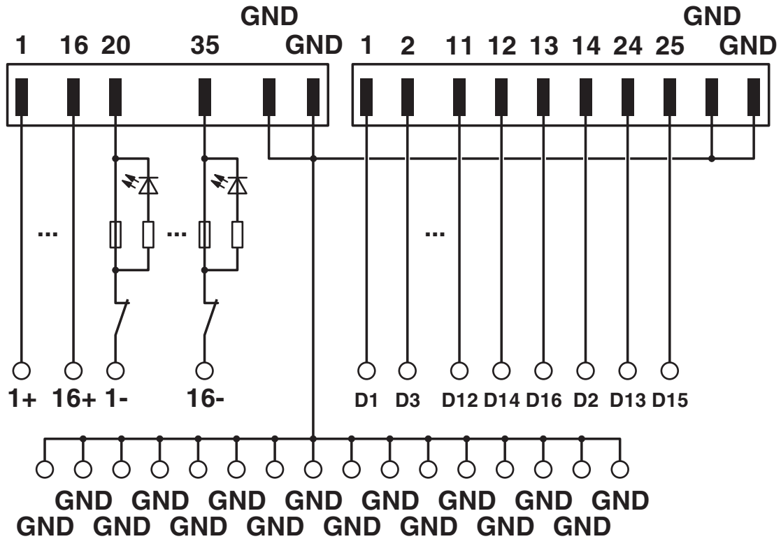
Diagrama eléctrico
