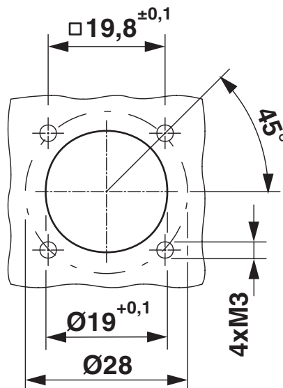
Dessin coté
