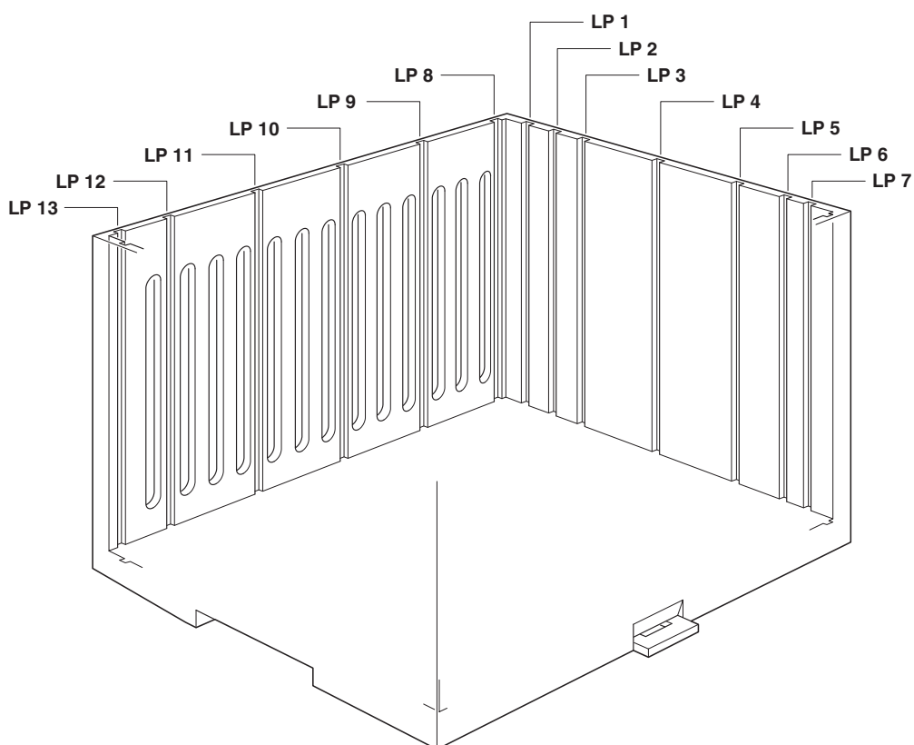
Plano esquemático
