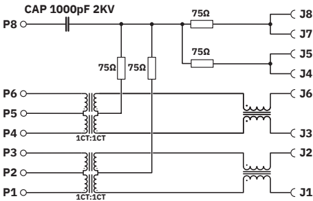
Schaltplan
