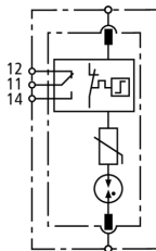
Schema di principio DG S 385 VA FM
