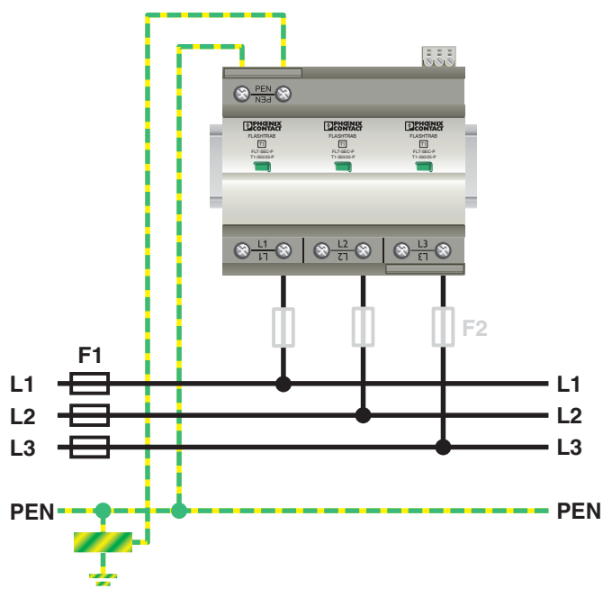
Applikationszeichnung
