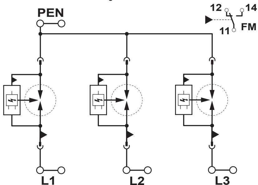
Diagrama eléctrico
