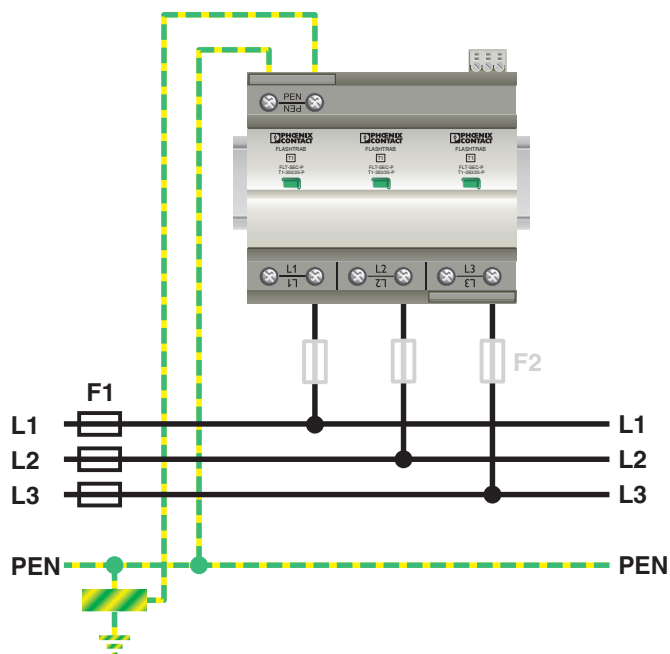
Dibujo de aplicación
