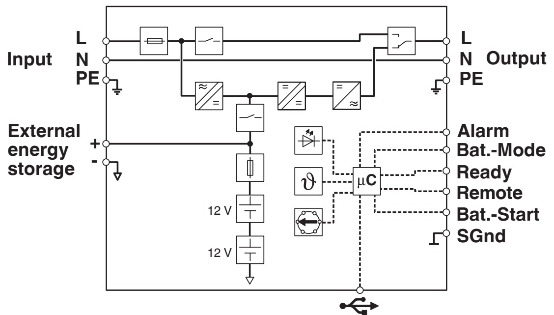
Blockschaltbild
