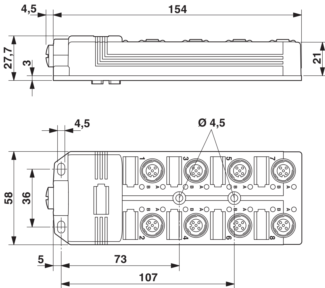
Dessin coté
