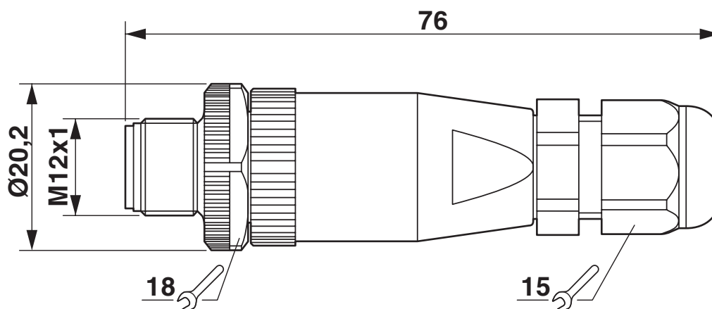
Maßzeichnung
