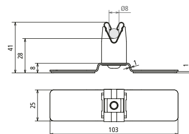
Maßbild DLH DG 8 H20 KP V2A AL
