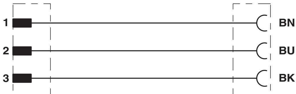
Diagrama eléctrico
