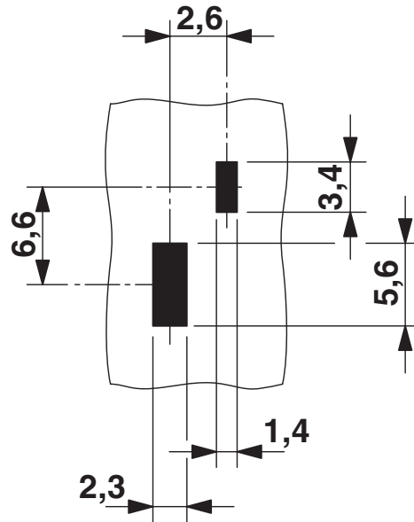
Bohrplan/Lötpadgeometrie
