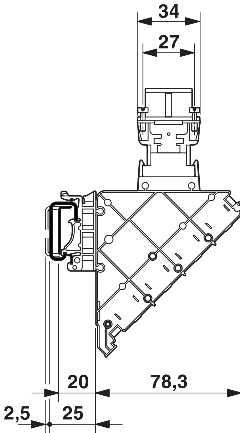
Maßzeichnung
