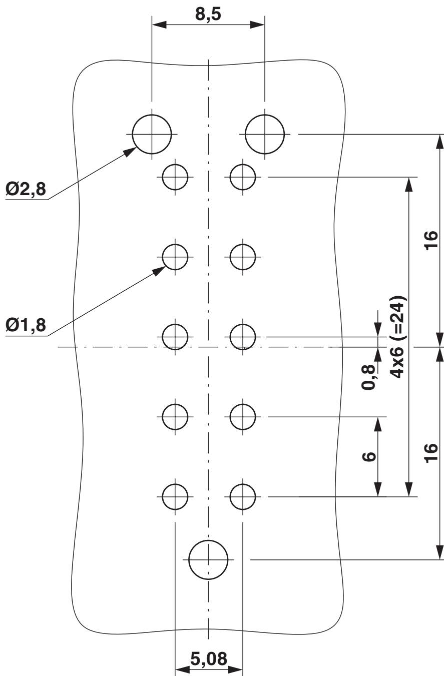
Gabarit perçage / géom. pastille soudage
