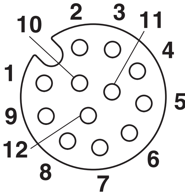
Dessin schématique
