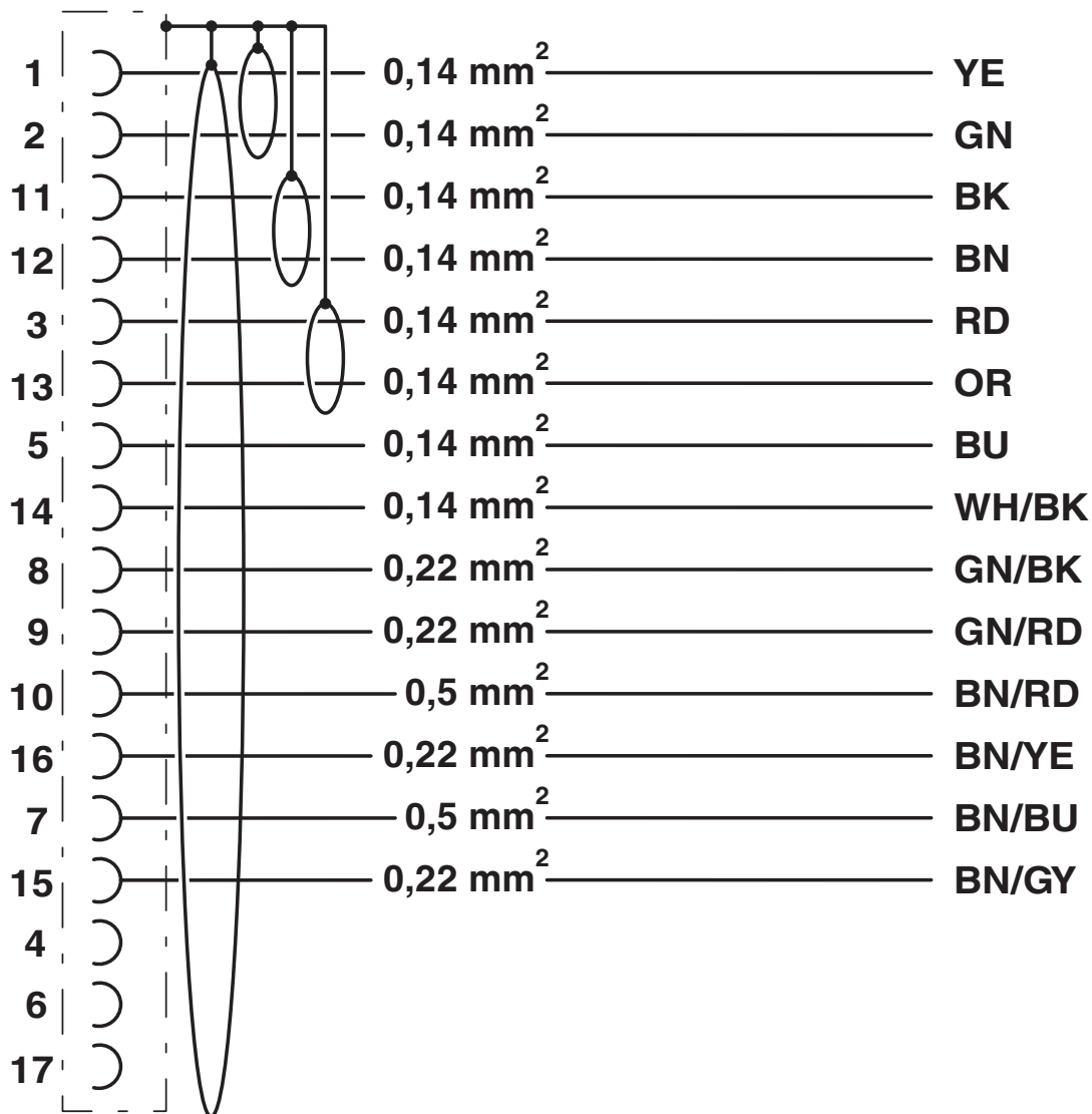
Diagrama eléctrico
