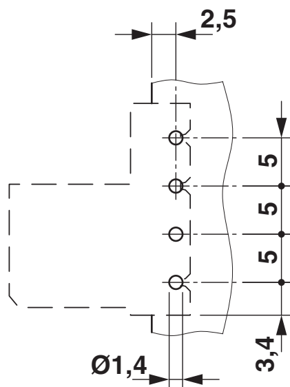
Bohrplan/Lötpadgeometrie
