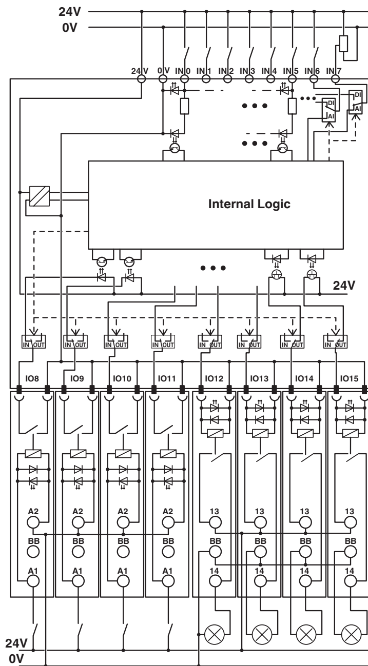
Schaltplan
