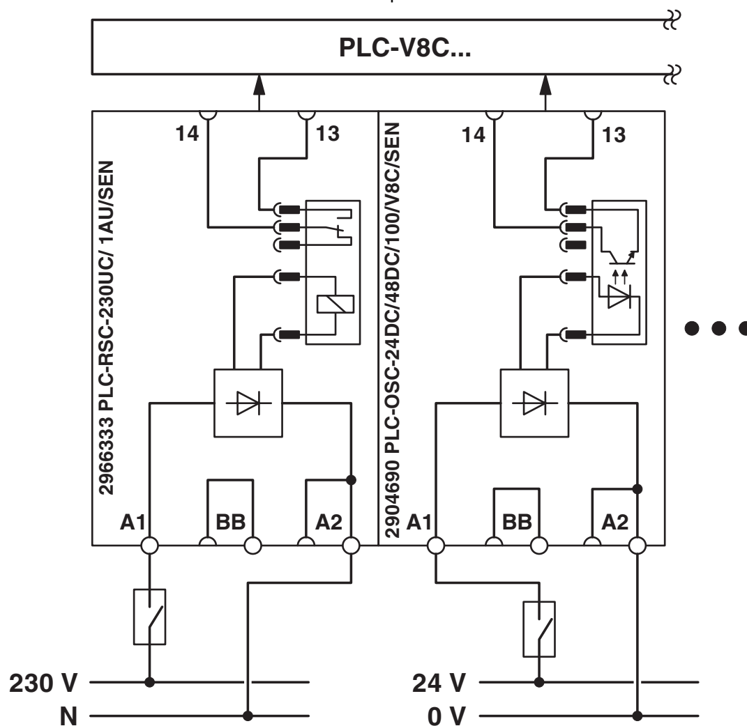
Schaltplan
