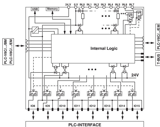
Diagrama eléctrico
