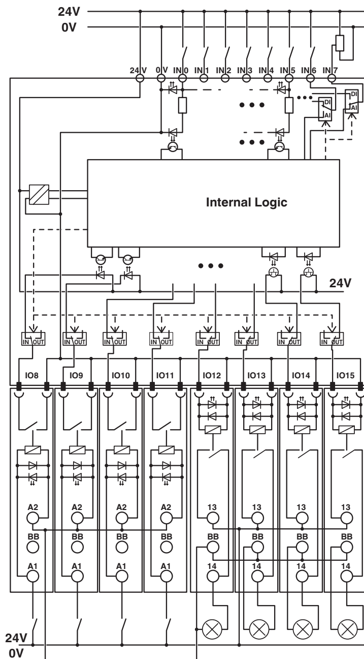
Diagrama eléctrico
