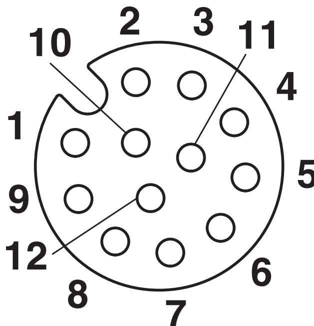
Plano esquemático
