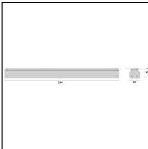
310424 Einbaugehäuse L 1094 mm
