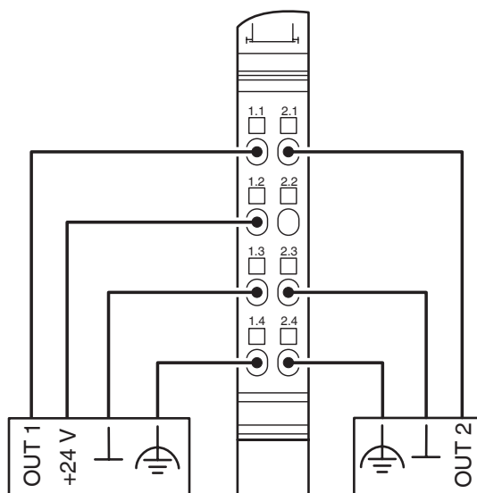
Dibujo de conexión
