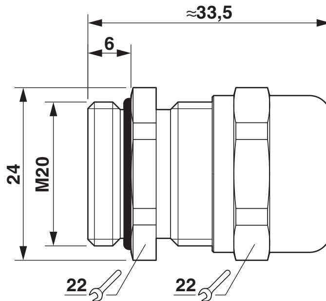
Maßzeichnung
