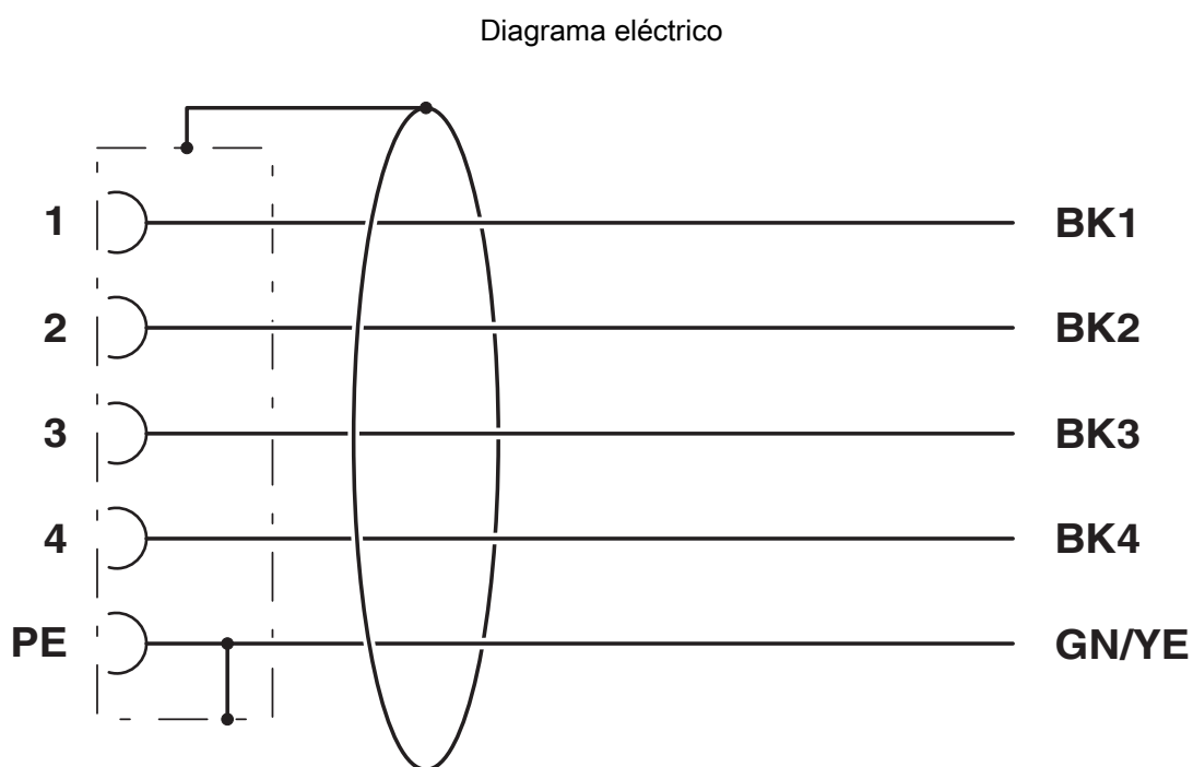
Ocupación de contactos del conector hembra M12
