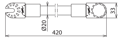
Maßbild ISV 420 ZK MS
