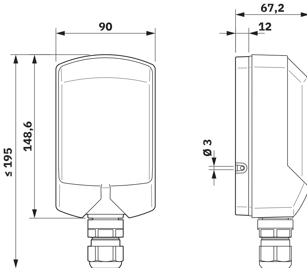
Dessin coté
