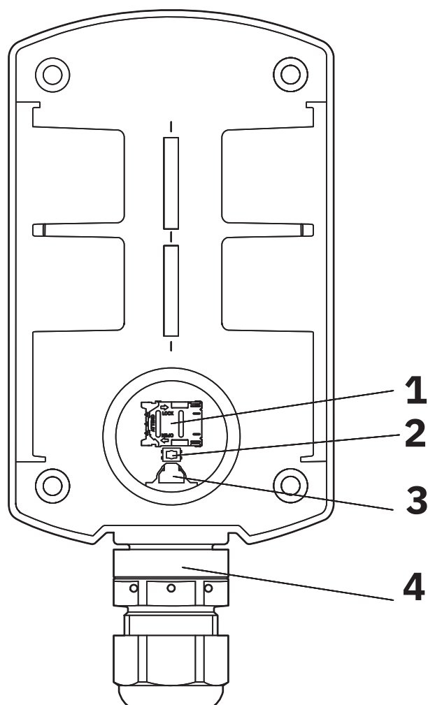
Dessin schématique
