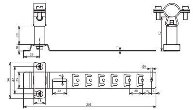
Maßbild DLH ZS 20 23 H55 L205 V2A
