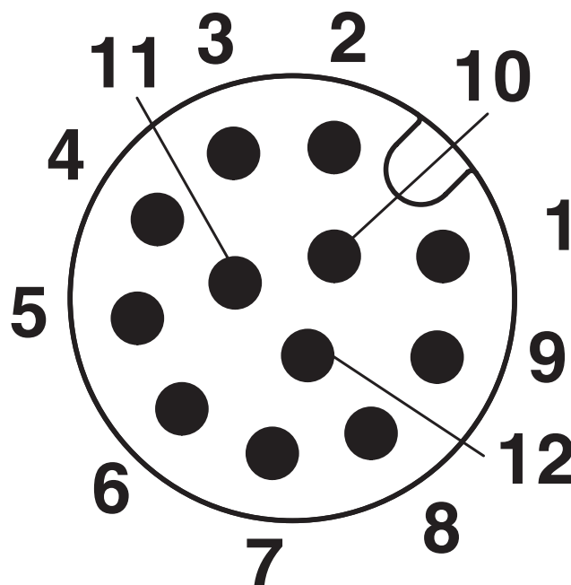
Plano esquemático
