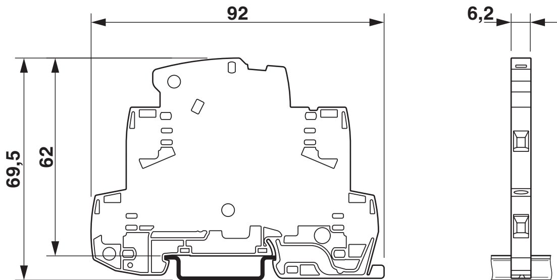
Dessin coté
