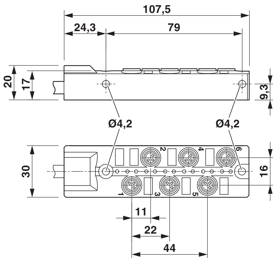
Dessin coté
