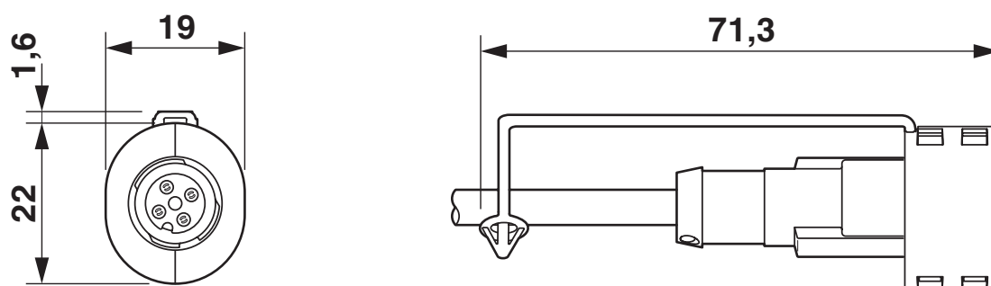
Connecteur femelle montée avec EXCLIP
