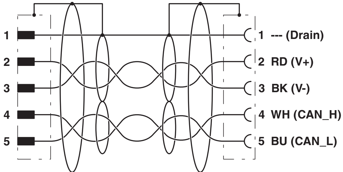
Diagrama eléctrico
