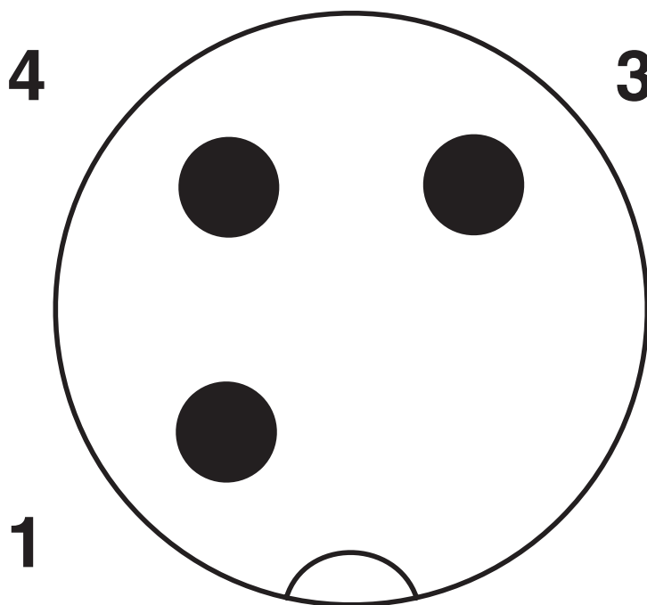
Plano esquemático
