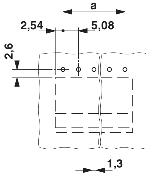
Bohrplan/Lötpadgeometrie
