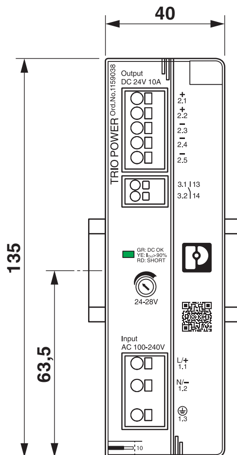
Maßzeichnung
