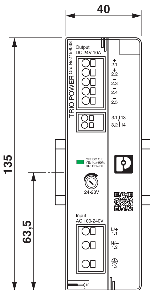
Esquema de dimensiones
