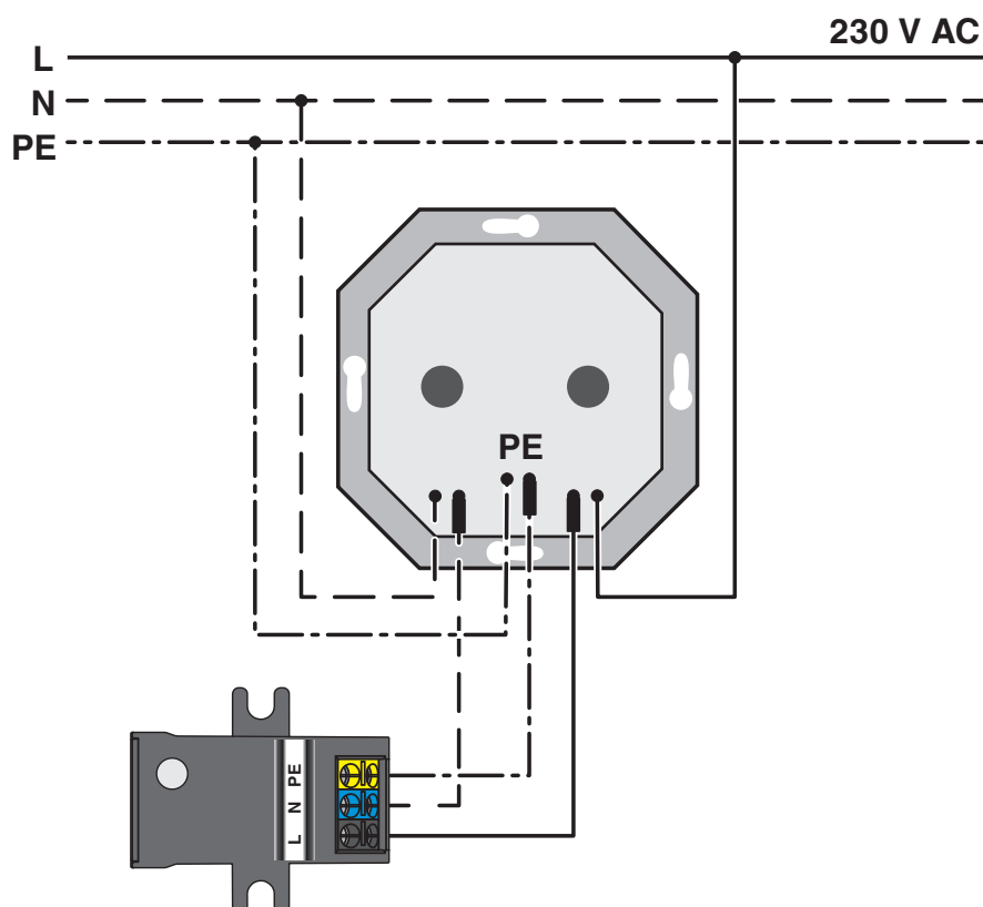
Applikationszeichnung
