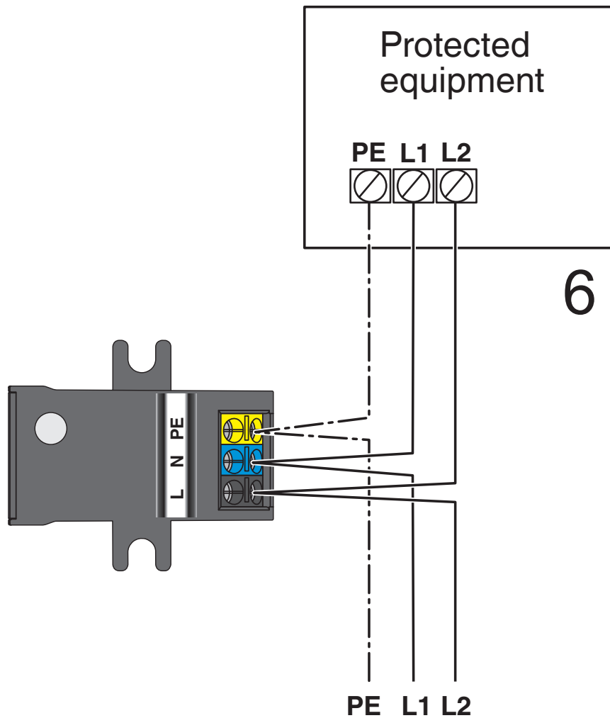
Applikationszeichnung
