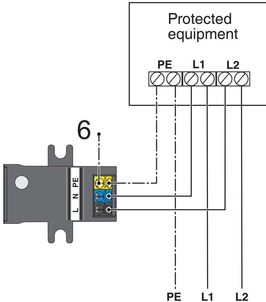
Applikationszeichnung
