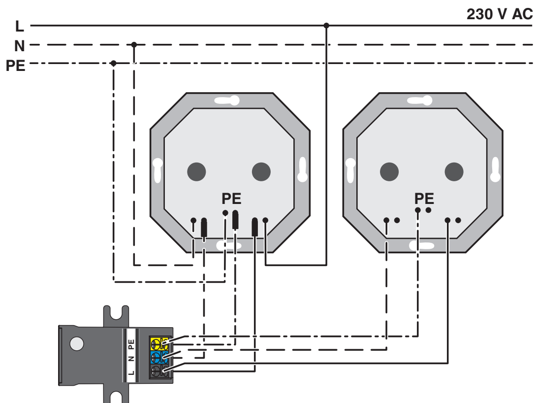
Applikationszeichnung
