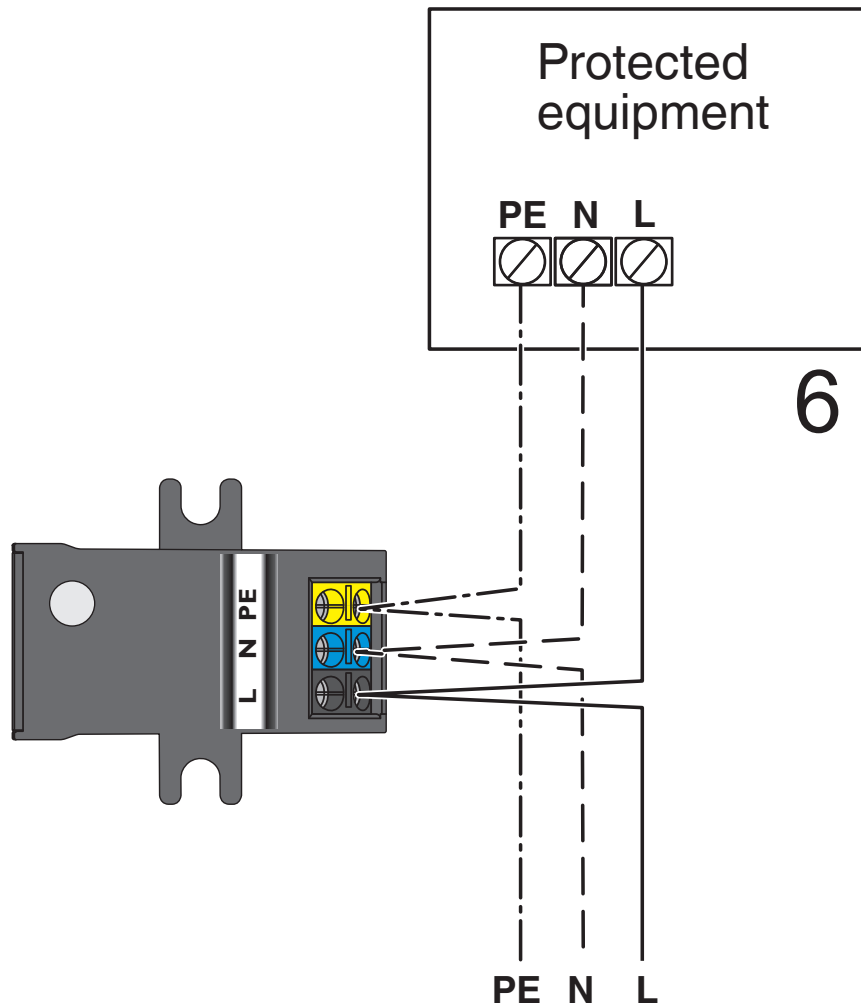
Applikationszeichnung
