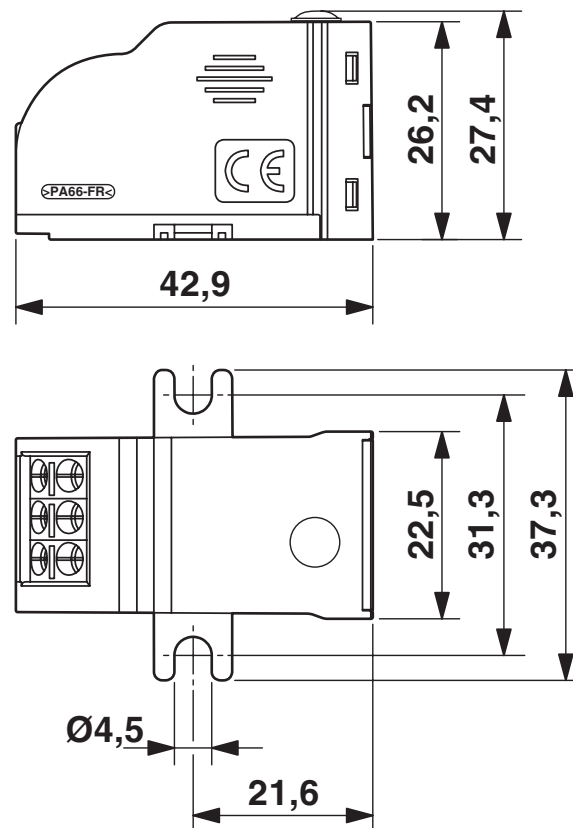
Dessin coté
